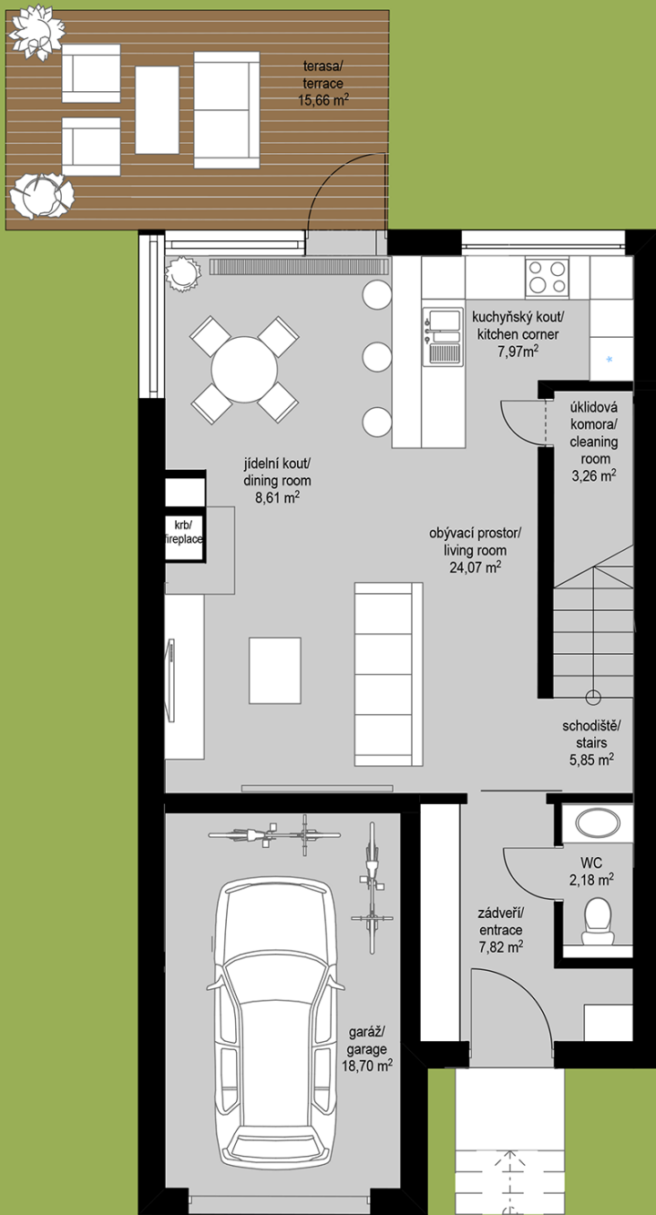
PŘÍZEMÍ/GROUND FLOOR
