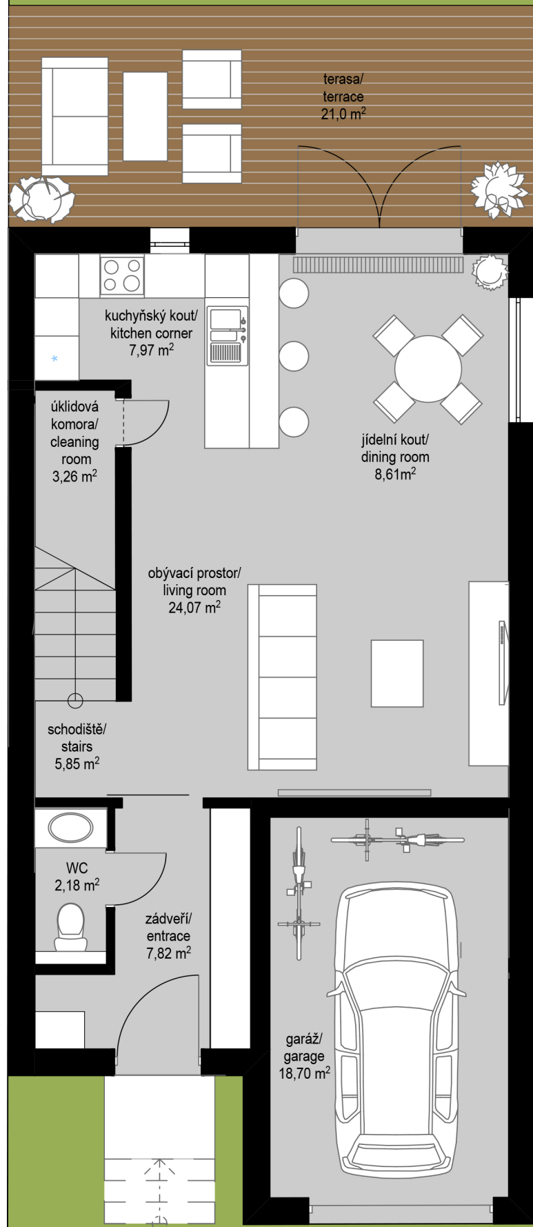
PŘÍZEMÍ/GROUND FLOOR
