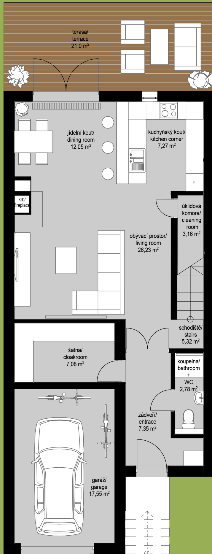
PŘÍZEMÍ/GROUND FLOOR
